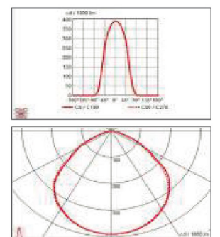
Lichtverteilungsdiagramm
