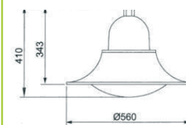
Abmessungen (mm)
